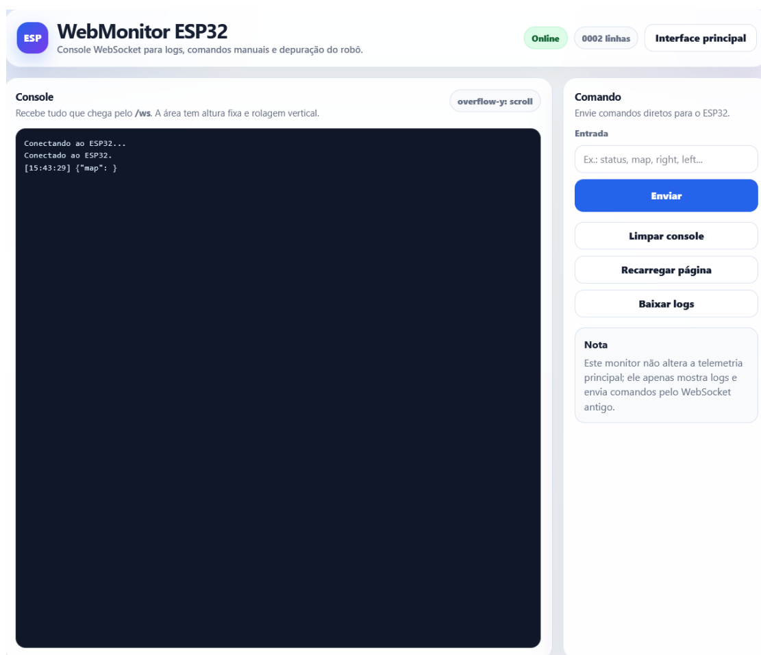
Figura 17 – Interface de monitoramento e logs em tempo real.
