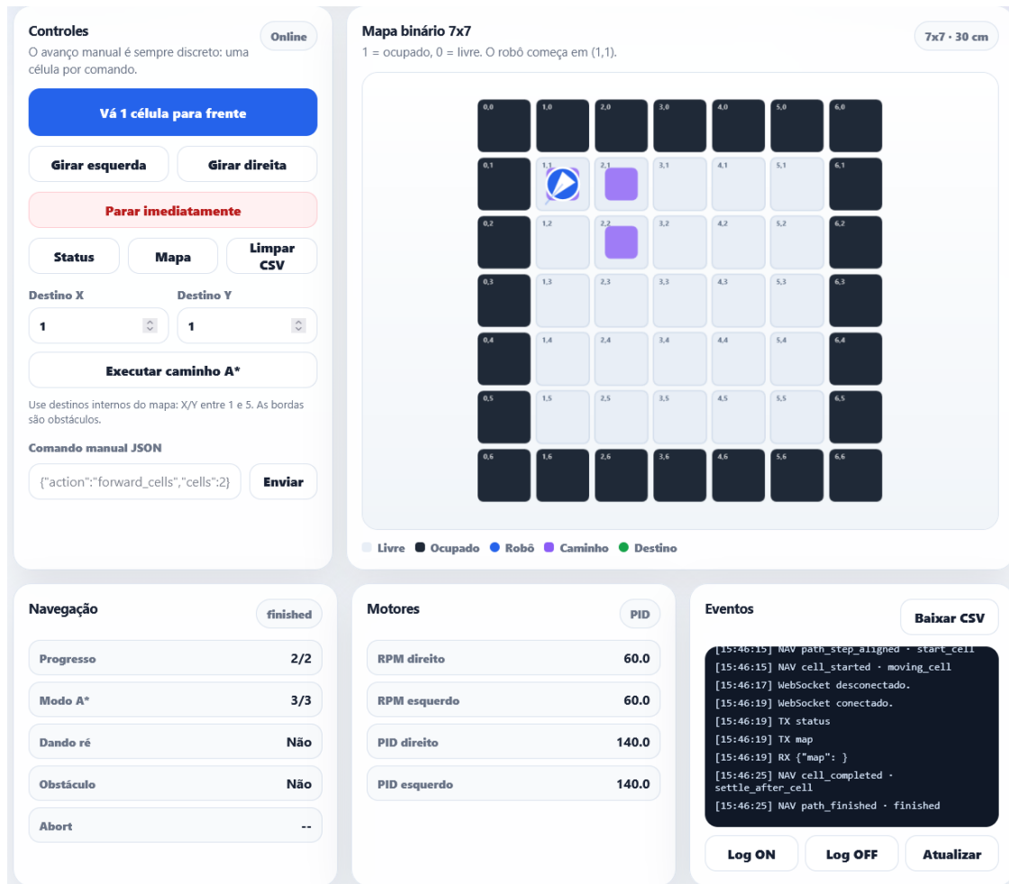
Figura 16 – Interface principal de controle do robô durante os testes.
