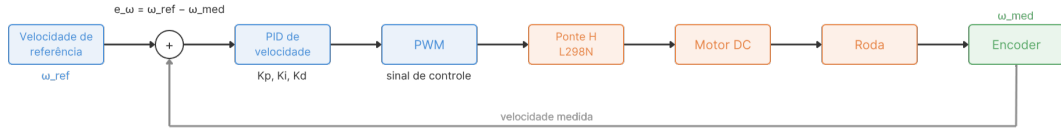
Figura 9 – Diagrama simplificado da malha de controle de velocidade dos motores.
