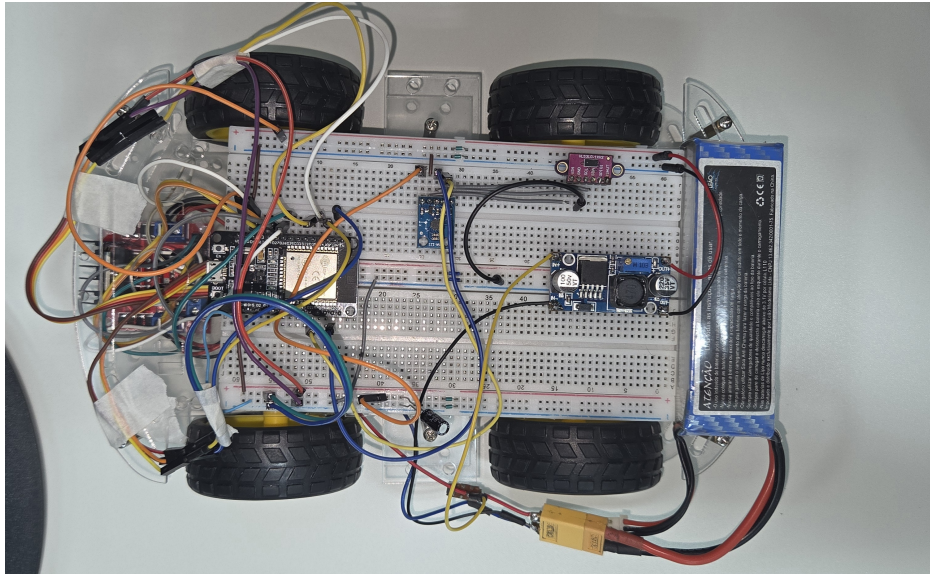
Figura 13 – Vista superior do protótipo final montado.
